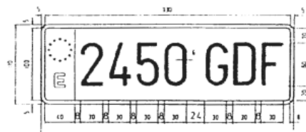
MATRÍCULA VEHÍCULOS AUTOMÓVILES ORDINARIA LARGA DEL ANTEPIÉ FONDO BLANCO CARACTERES NEGRO MATE
